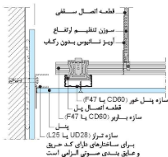
اتصال به دیوار پوششی W611
