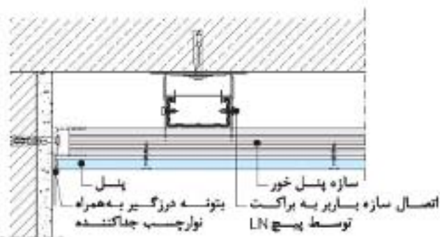
اتصال به دیوار بتایی
