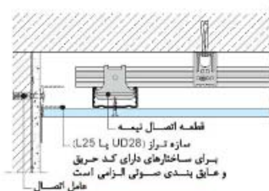
اتصال به دیوار بتایی
