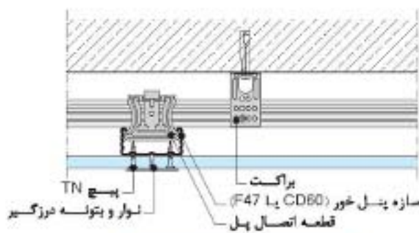
اتصال و درزگیری لبه پش خورده
