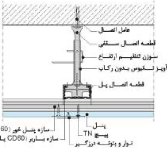
اتصال و درزگیری لبه طولی
