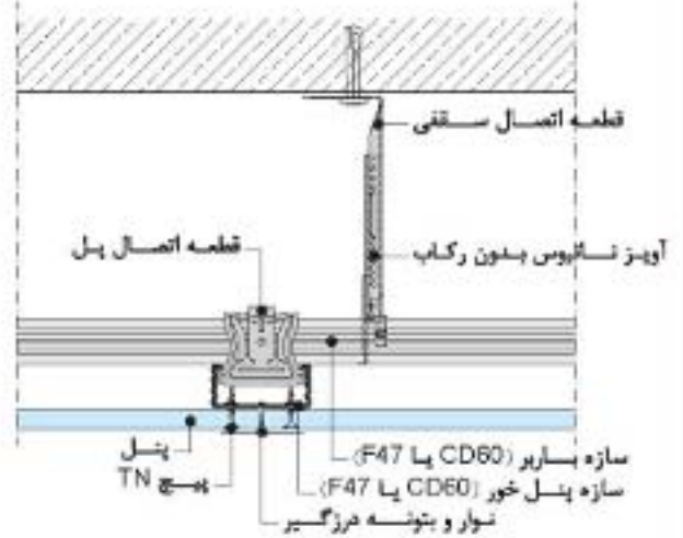
اتصال و درزگیری لبه برش خورده
