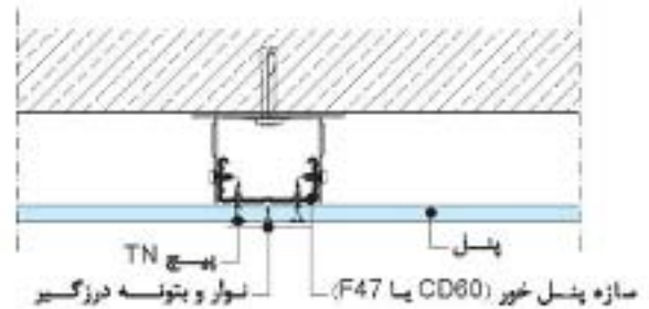
اتصال به دیوار بتنی
