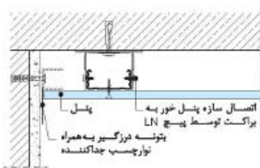
اتصال به دیوار بتنی
