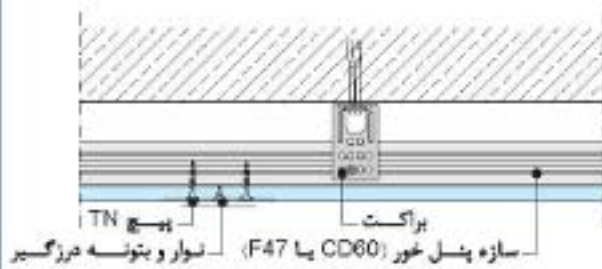
اتصال به دیوار بتنی
