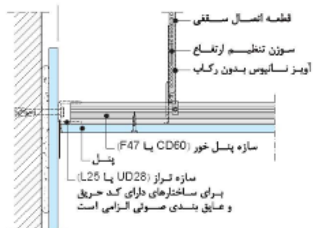
اتصال به دیوار پوششی W611
