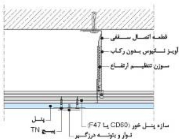
اتصال و درزگیری لبه طولی
