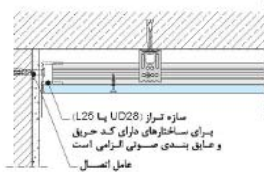
اتصال به دیوار بتنی
